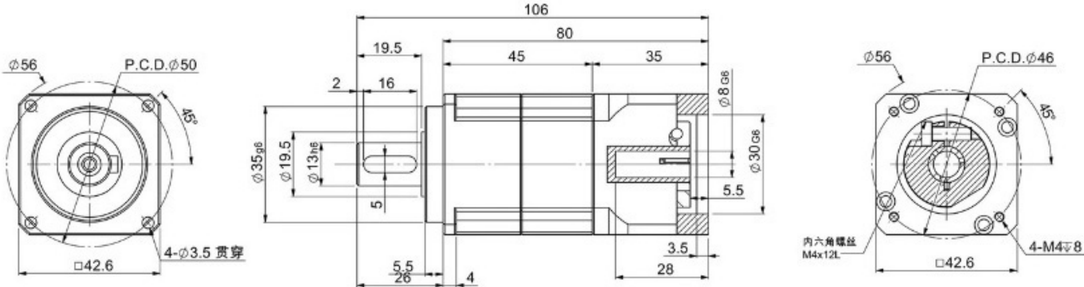
Level 2 speed ratio drawings (20:1 25:1 35:1 40:1 50:1 70:1 100:1)
